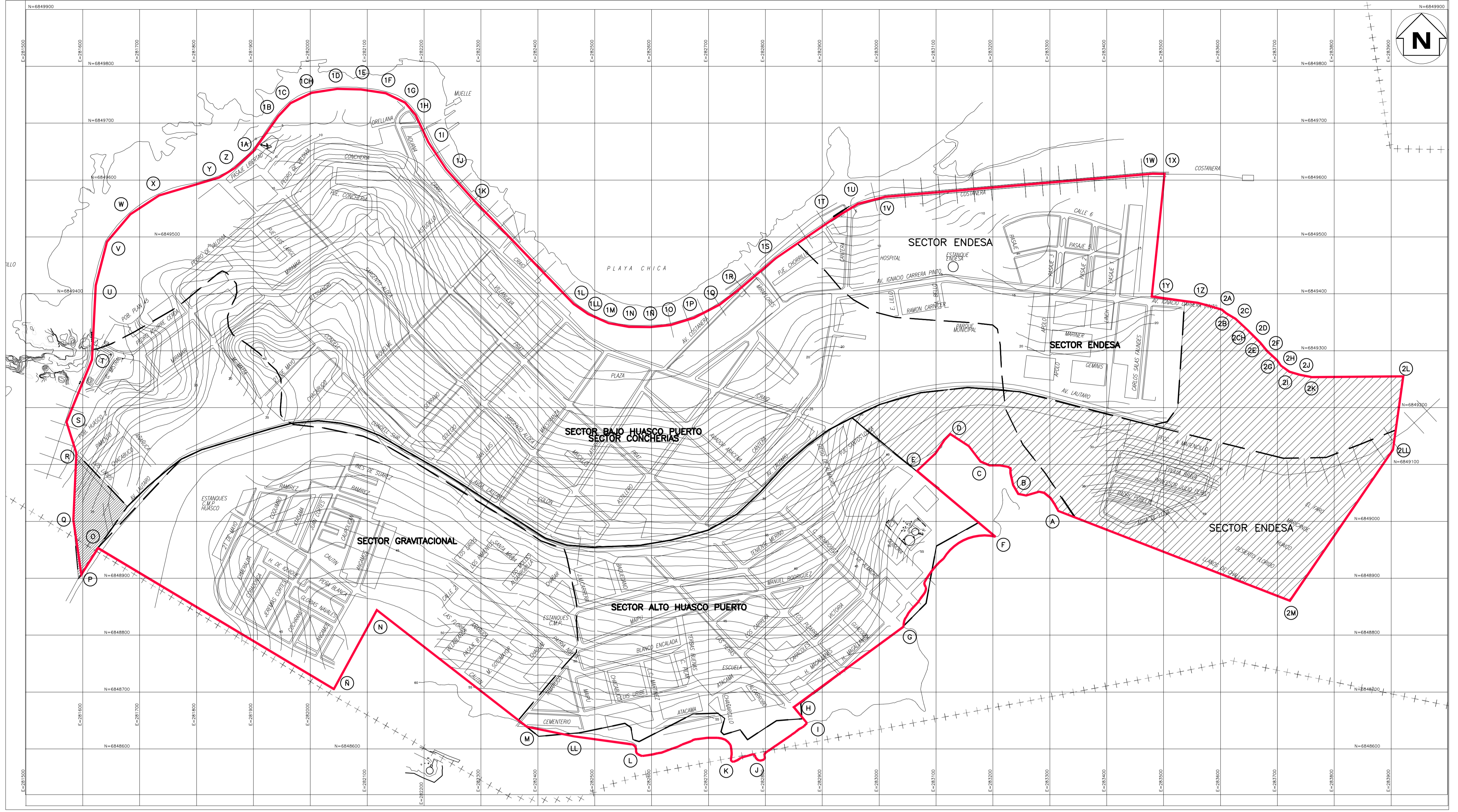
PLANTA GENERAL DE HUASCO PUERTO TERRITORIO OPERACIONAL ESCALA 1:4.000
